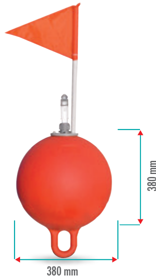
M03430 26 LT BAYRAKLI KÜRE ŞAMANDIRA Yüzdürmesi : 25 kg Ürün Ağırlığı: 1,2 kg
