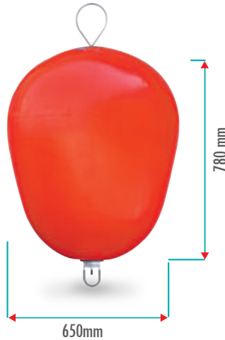
M03091 170 LT ŞAMANDIRA Yüzdürmesi : 155 kg Ürün Ağırlığı: 18 kg
