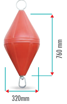
M03200 17 LT ŞAMANDIRA Yüzdürmesi : 15 kg Ürün Ağırlığı: 2,7 kg
