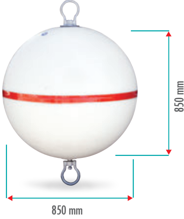
M03325 320 LT ŞAMANDIRA Yüzdürmesi : 290 kg Ürün Ağırlığı: 30 kg
