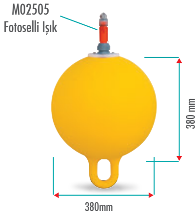
M03410 26 LT FENERLİ KÜRE ŞAMANDIRA Yüzdürmesi : 25 kg Ürün Ağırlığı: 1,2 kg
