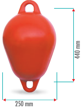
M03100 9 LT ARMUT ŞAMANDIRA Yüzdürmesi : 8 kg Ürün Ağırlığı: 650 gr
