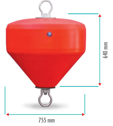
M03345 200 LT ŞAMANDIRA Yüzdürmesi : 180 kg Ürün Ağırlığı: 17 kg
