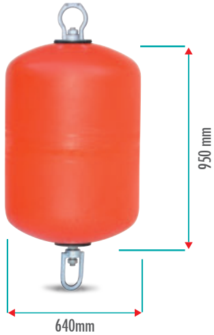
M03340 200 LT ŞAMANDIRA Yüzdürmesi : 180 kg Ürün Ağırlığı: 22 kg
