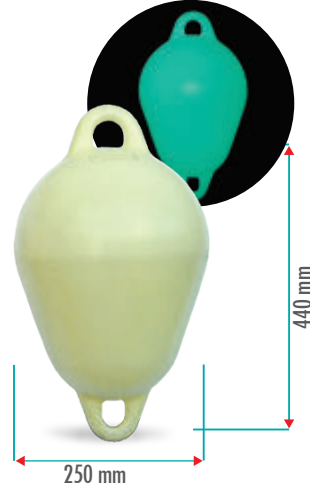
M03110 9 LT FOSFORLU ARMUT ŞAMANDIRA Yüzdürmesi : 8 kg Ürün Ağırlığı: 650 gr Not: Gündüz aldığı ışığı gece yansıtma özelliğine sahiptir.
