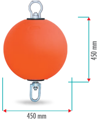
M03360 50 LT ŞAMANDIRA Yüzdürmesi : 35 kg Ürün Ağırlığı: 4 kg
