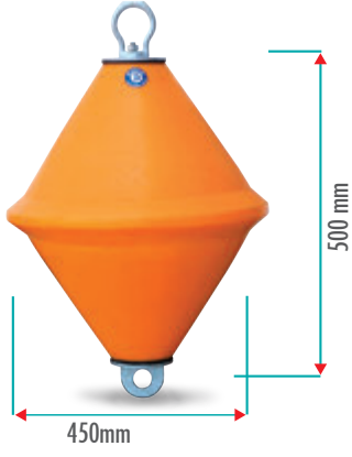
M03205 30 LT ŞAMANDIRA Yüzdürmesi : 20 kg Ürün Ağırlığı: 4 kg
