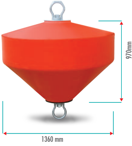
M03305 900 LT ŞAMANDIRA Yüzdürmesi : 800 kg Ürün Ağırlığı: 65 kg
