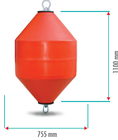
M03330 300 LT ŞAMANDIRA Yüzdürmesi : 250 kg Ürün Ağırlığı: 28 kg
