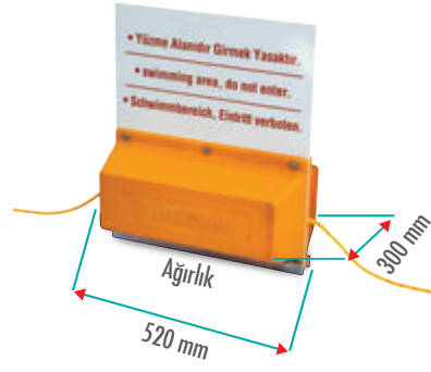
M03252 UYARI LEVHASI
