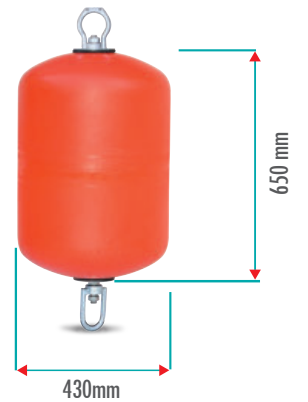
M03350 100 LT ŞAMANDIRA Yüzdürmesi : 90 kg Ürün Ağırlığı: 11 kg
