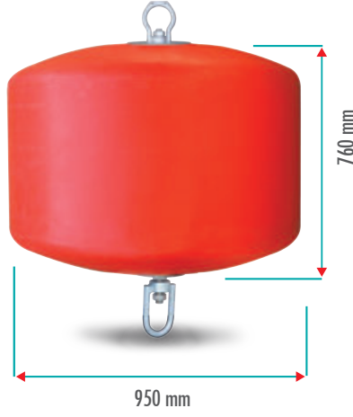
M03310 600 LT ŞAMANDIRA Yüzdürmesi : 500 kg Ürün Ağırlığı: 60 kg
