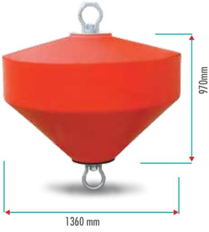
M03305 900 LT ŞAMANDIRA / BUOY Yüzdürmesi / Buoyancy: 800 kg Ürün Ağırlığı / Weight: 65 kg
