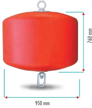
M03310 600 LT ŞAMANDIRA / BUOY Yüzdürmesi / Buoyancy: 500 kg Ürün Ağırlığı / Weight: 60 kg
