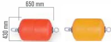
M03523 100 LT Ağırlık / Weight: 11 kg Yüzdürme / Buoyancy: 90 kg
