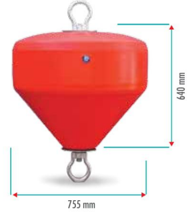
M03345 200 LT ŞAMANDIRA / BUOY Yüzdürmesi / Buoyancy: 180 kg Ürün Ağırlığı / Weight: 17 kg
