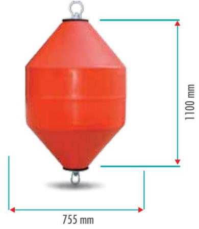
M03330 300 LT ŞAMANDIRA / BUOY Yüzdürmesi / Buoyancy: 250 kg Ürün Ağırlığı / Weight: 28 kg
